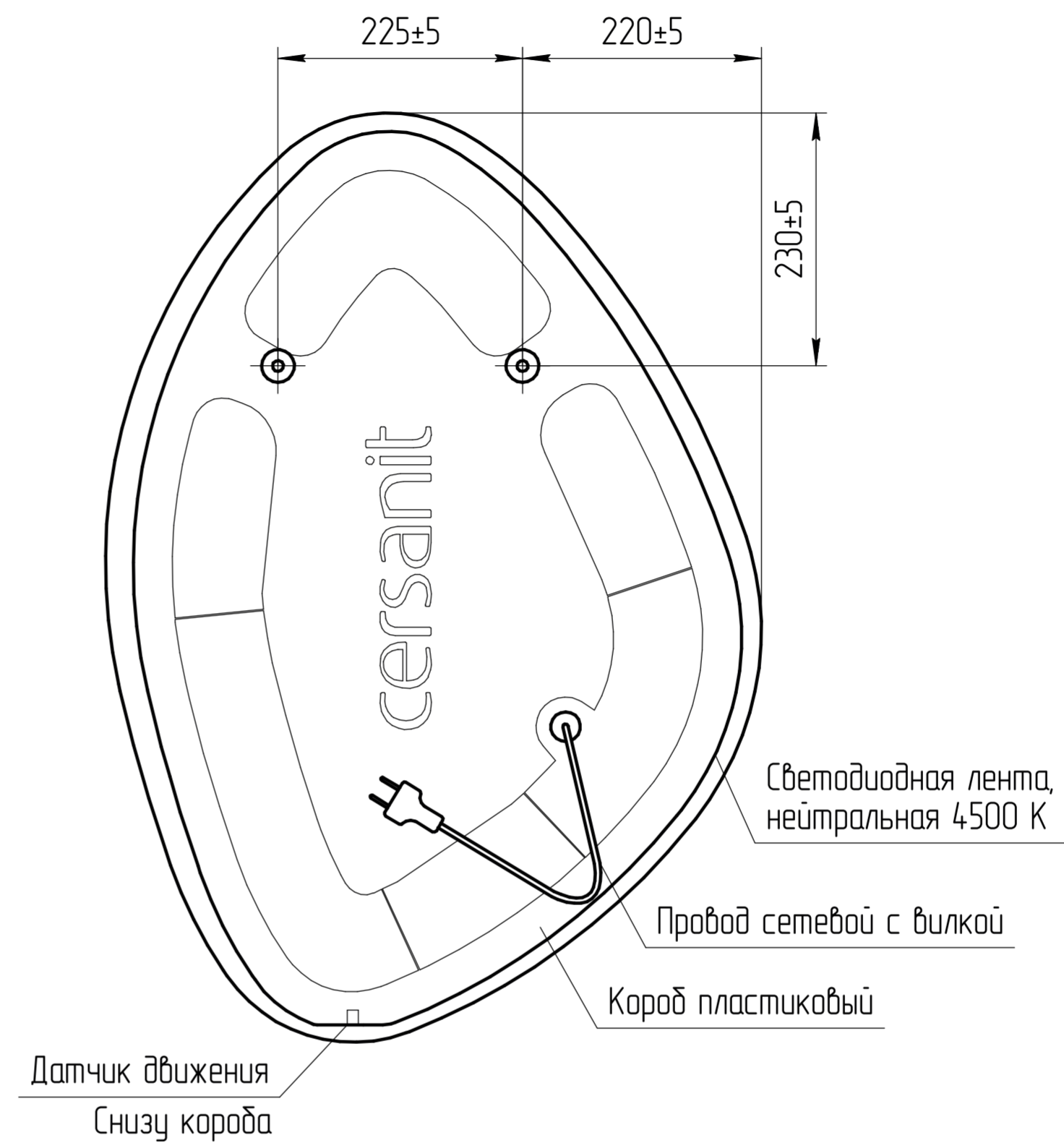
Вид сзади (М 1:5)
