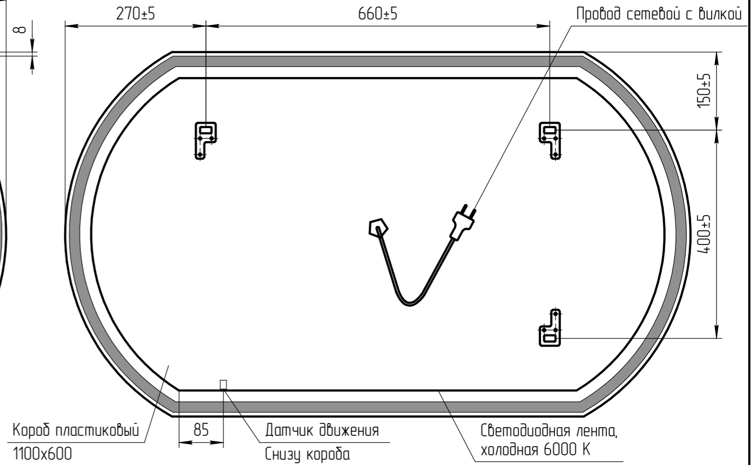
Вид сзади (М 1:5)
