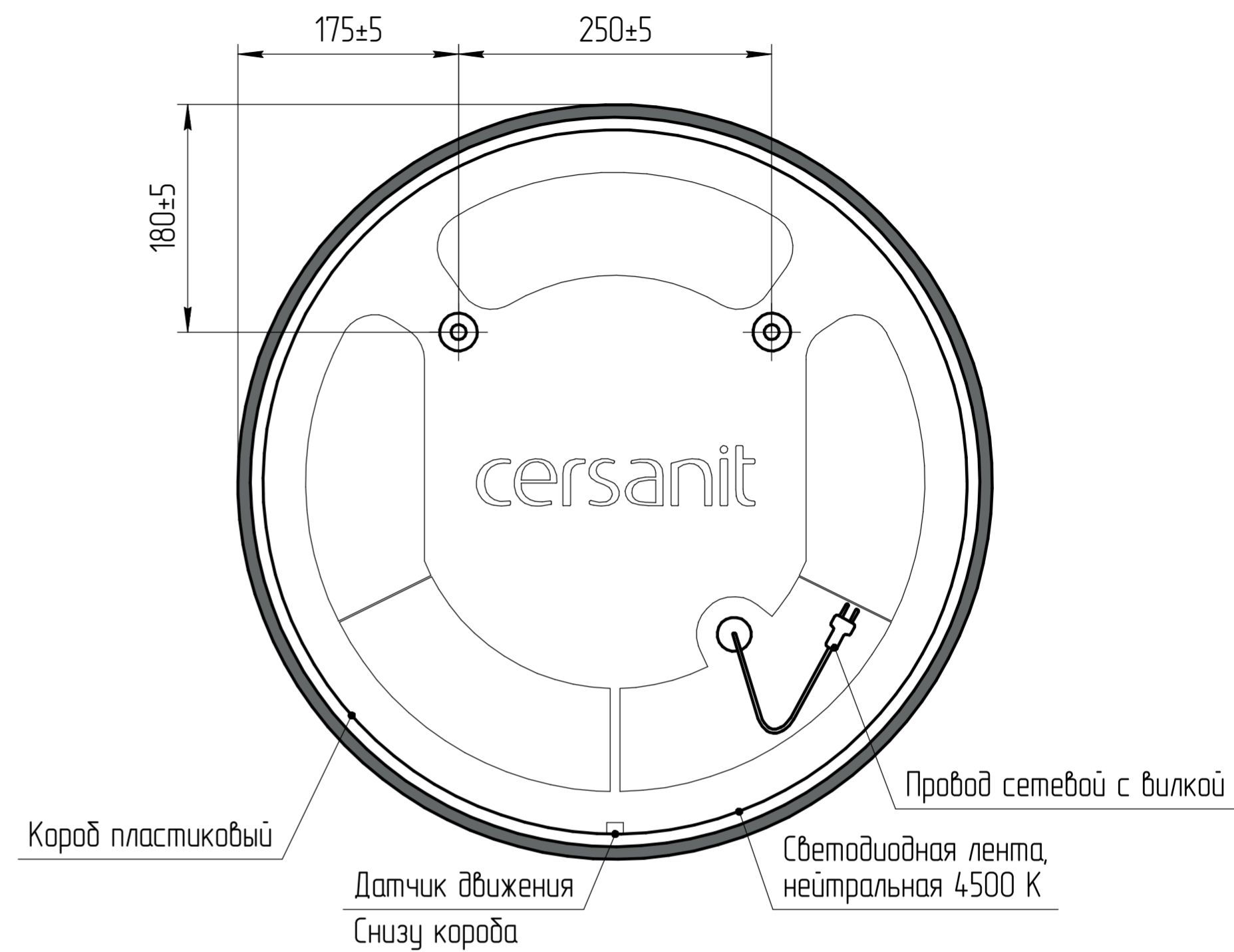
Вид сзади (М 1:4)
