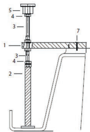
Рис.4: Схема сборки дополнительных ножек (поз. C на рис.1) (цифрами отмечены номера деталей)
