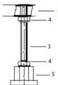
Рис.3: Схема сборки дополнительных ножек (поз. D на рис.1) (цифрами отмечены номера деталей)
